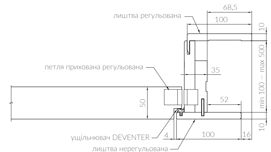
Монтаж плоских дверей з коробкою Smart Reverse
