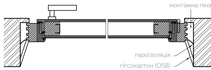
Стіна без чверті. З відкосом
