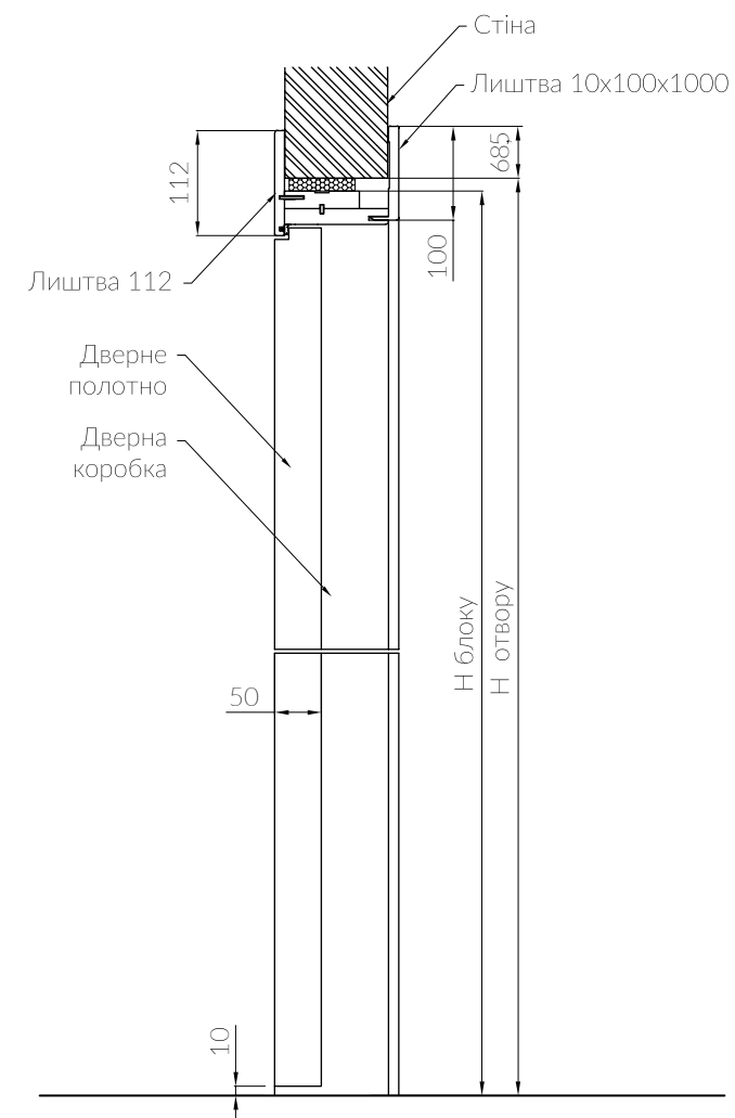
Монтаж плоских дверей з коробкою Smart Reverse
