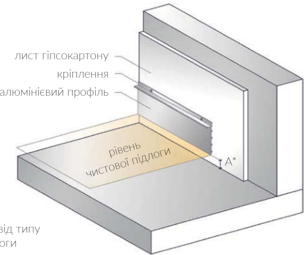
Підготовка до монтажу
