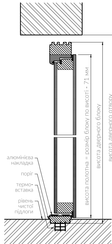
Вертикальний перетин
