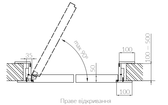
Стандартне відкривання на 90°
