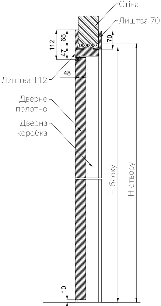
Відкриття Reverse на 90°
