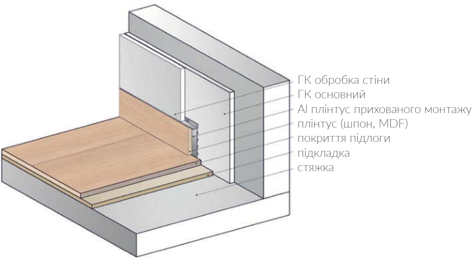
Змонтований плінтус
