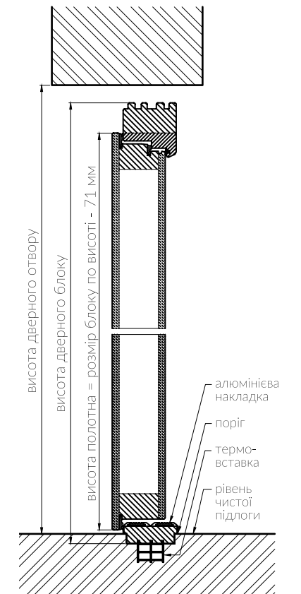
Вертикальний перетин
