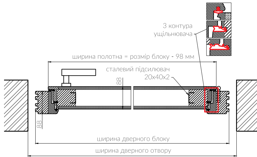
Горизонтальний перетин
