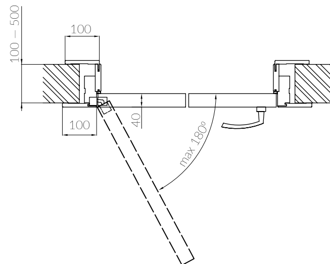
Стандартне відкривання на 180°
