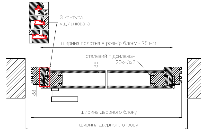
Горизонтальний перетин
