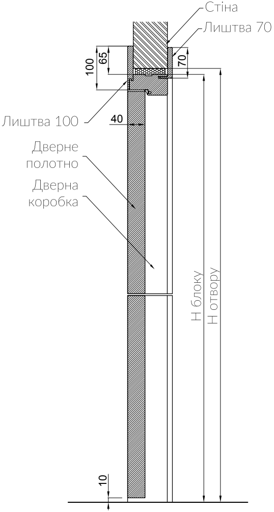
Стандартне відкриття на 180°
