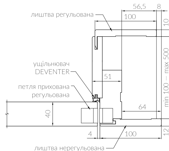
Монтаж плоских дверей з коробкою Smart
