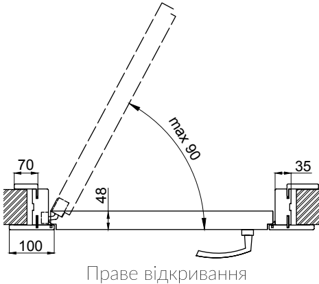
Відкриття Reverse на 90°
