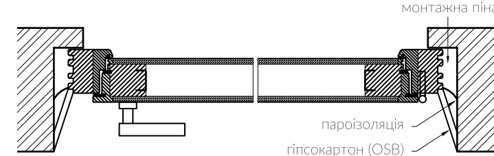
Стіна без чверті. З відкосом
