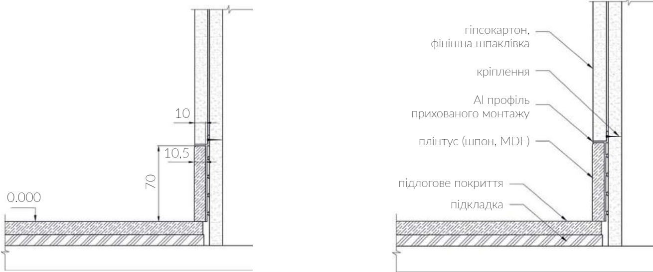
Розміри
